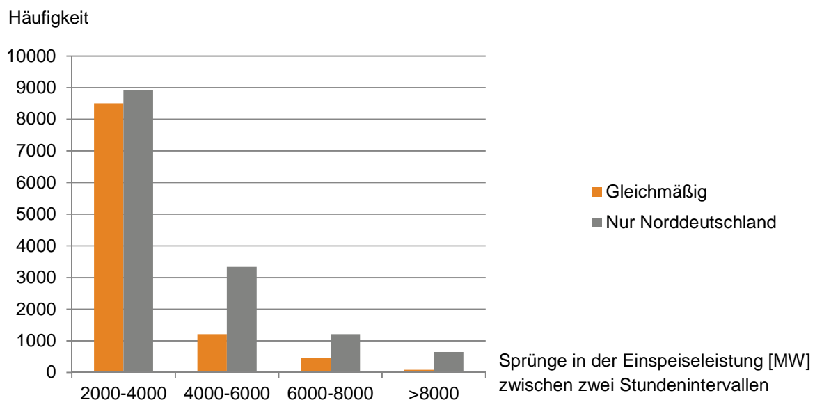
Abbildung 5: Anzahl und Höhe der Sprünge in der Einspeiseleistung zwischen zwei Stundenintervallen
